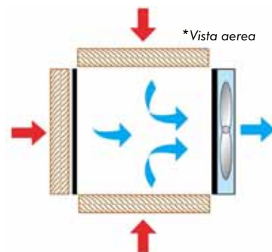
Principio de flujo de aire en el FCA 35 S (lateral) y abajo el FCA 35 B (inferior)
